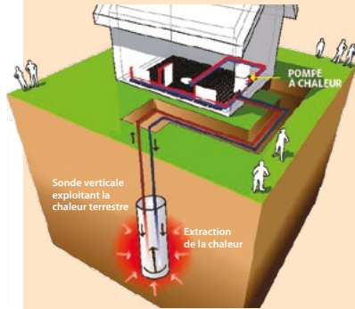
Illustration expliquant le principe de la géothermie. ©AFPG Association Française des Professionnels de la Géothermie
